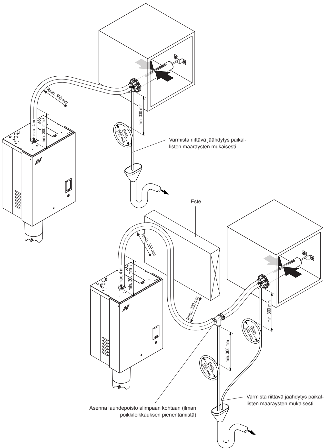
Kuva 19: Höyryjakoputki on asennettu alle 500 mm laitteen yläreunan ylä- tai alapuolelle.
