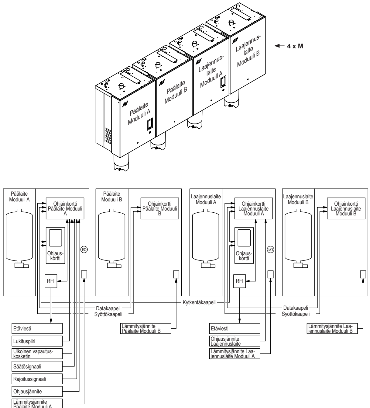
Kuva 5: Yhdistettyjen laitejärjestelmien yleiskuvaus (4 x "M")
