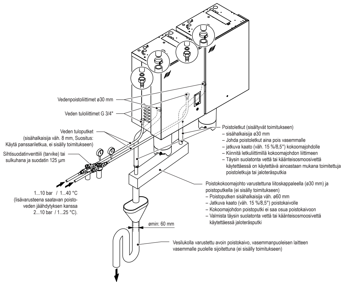
Kuva 24: Keskikokoisten ("M") kaksoislaitteiden vesiasennuksen yleiskuvaus
