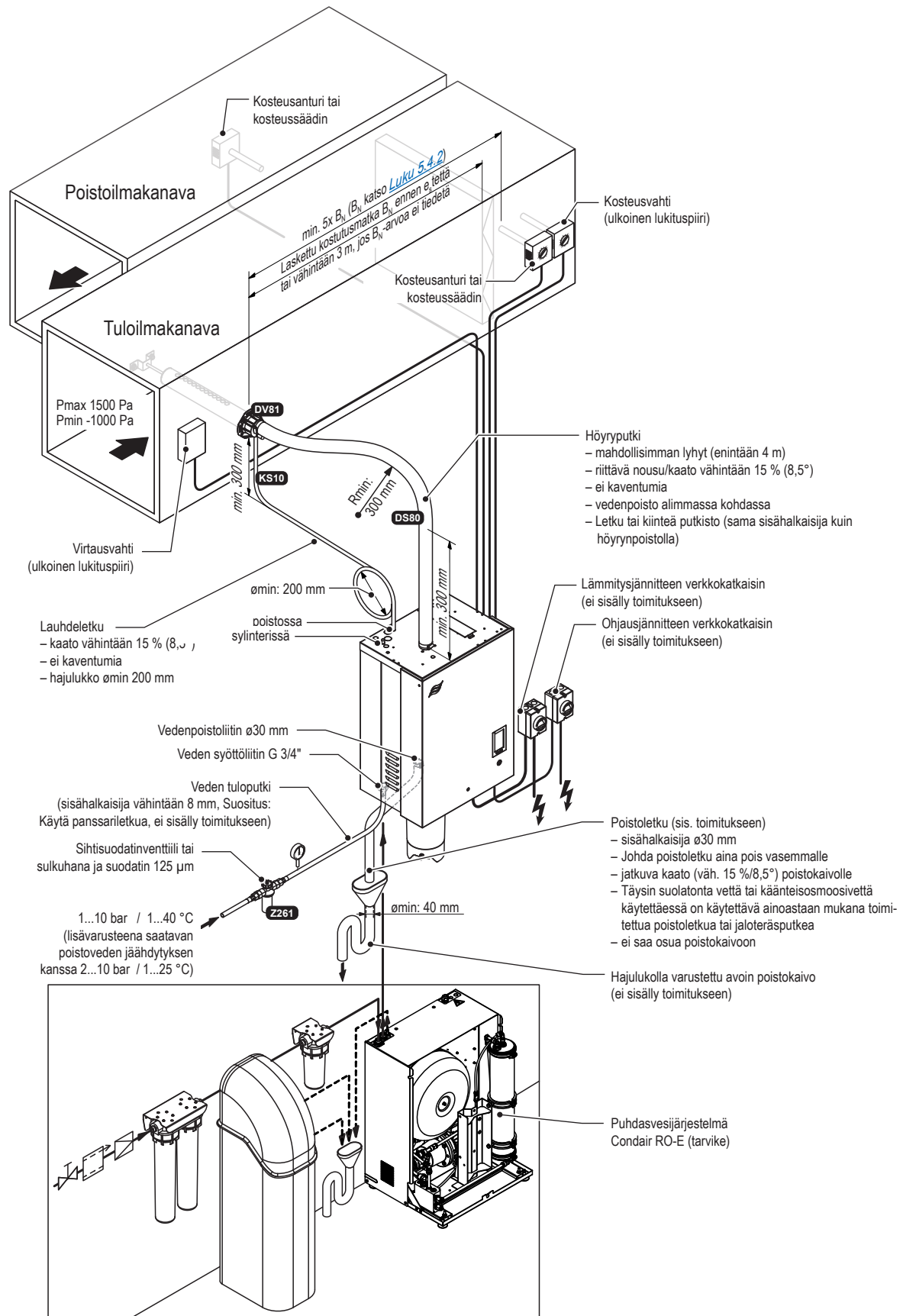
Kuva 8: Tyypillinen kanavakostutusasennus
