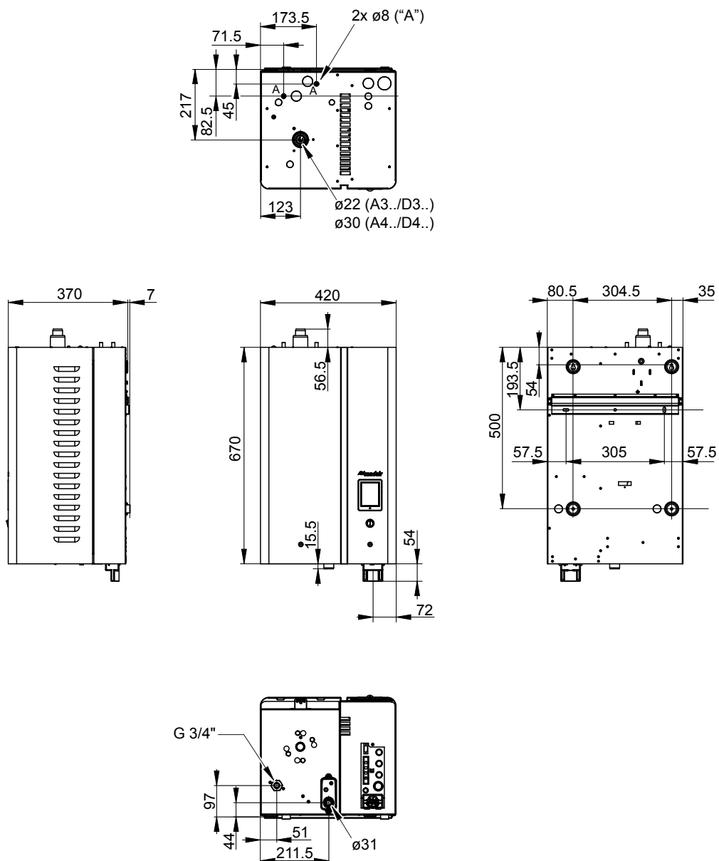
Kuva 31: Mittapiirustus Condair EL 5 - 15, kotelokoko "S" (mitat mm)
