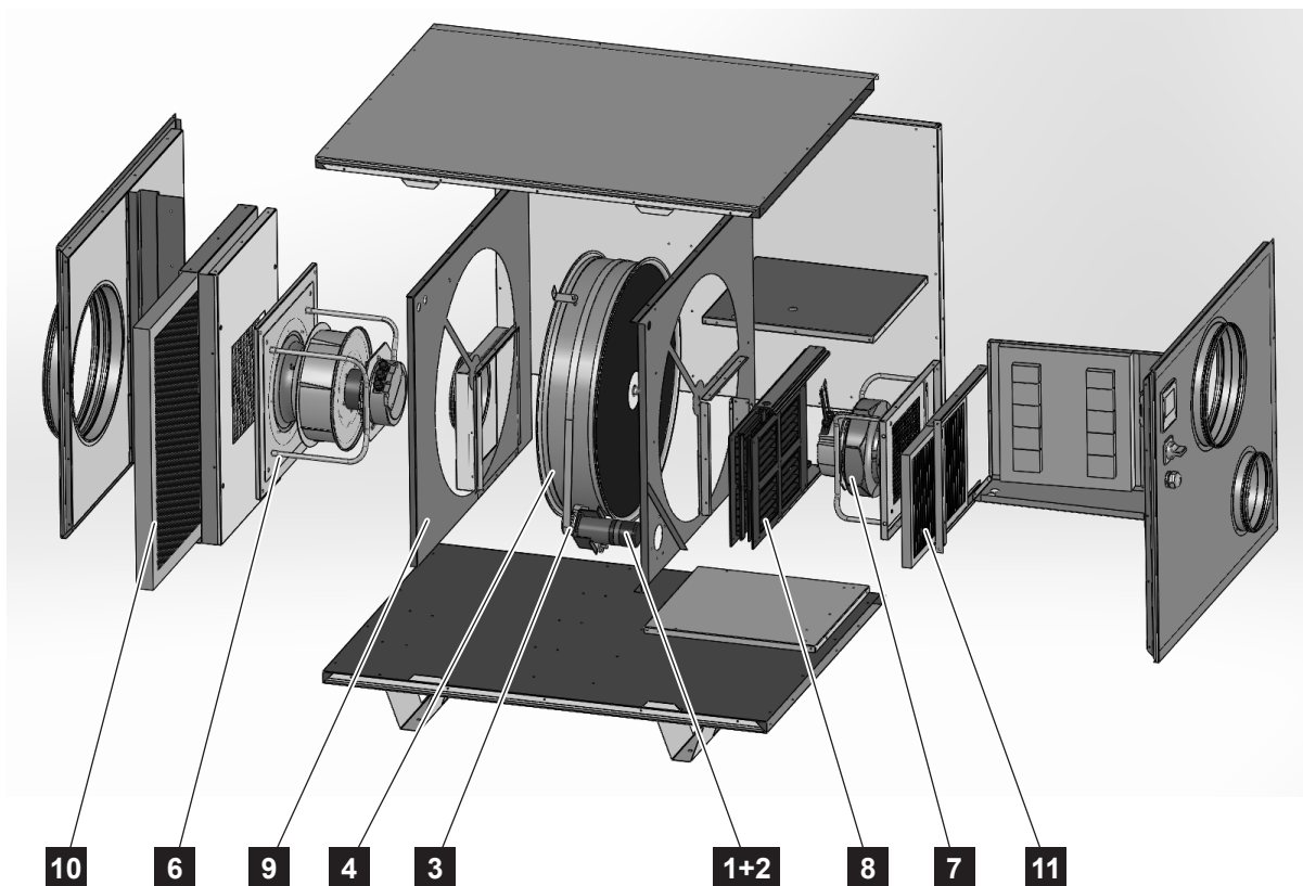
Kuva 5: Räjäytyskuva
