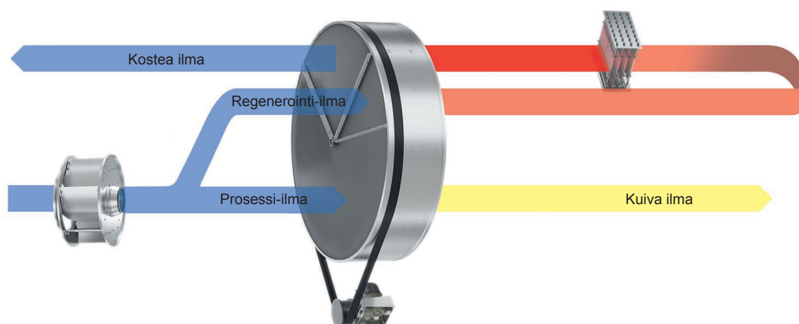
Kuva 2: Toimintaperiaate
