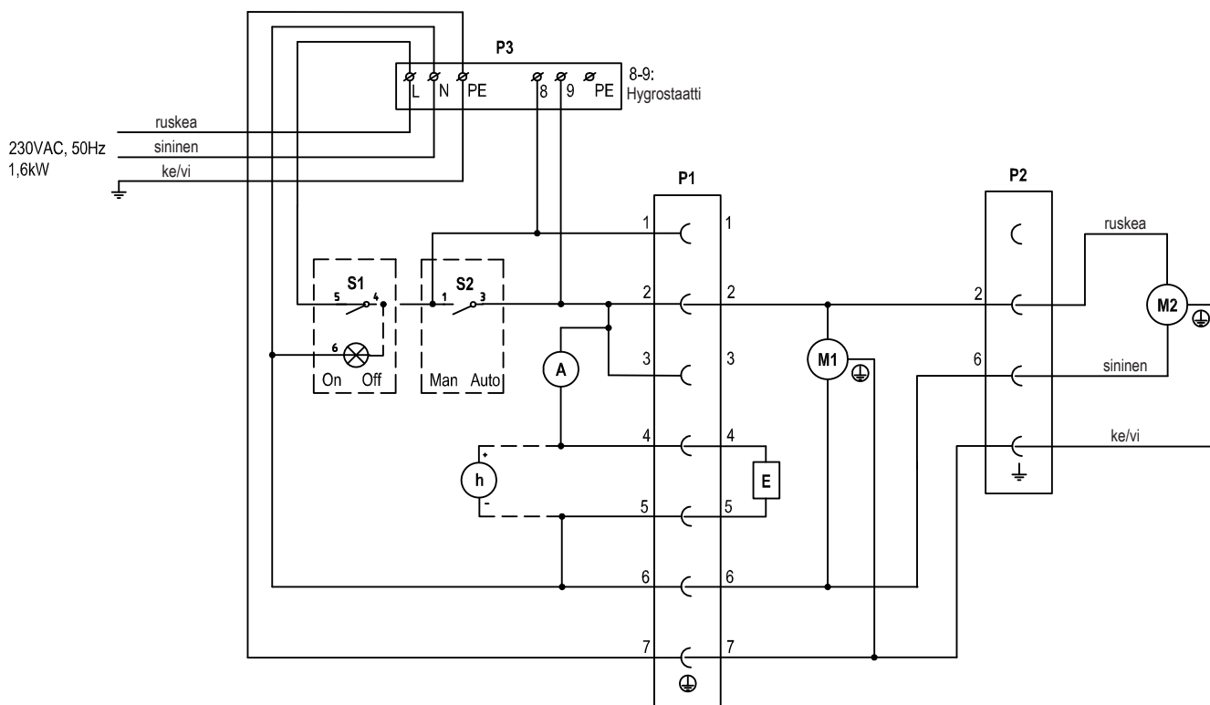
Kuva 6: Sähkökytkentä Condair DA 250
